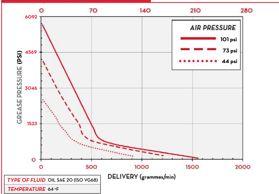
PIUSI P60:1 - 470
